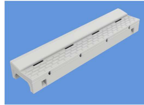
○乗入れB(20/20) 本体上部詳細図
