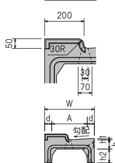
○乗入れD(50/50) 本体上部詳細図
